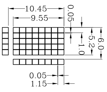
DETAIL DOTS SCALE: 2:1
